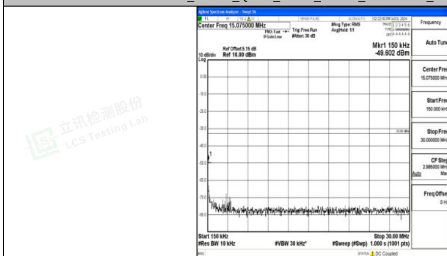
Band4 10MHz QPSK 20350 1RB#0 0.15~30 0.15~30
