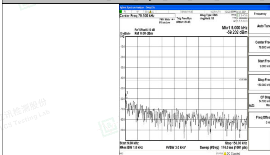
Band4 10MHz QPSK 20350 1RB#0 0.009~0.15 0.009~0.15
