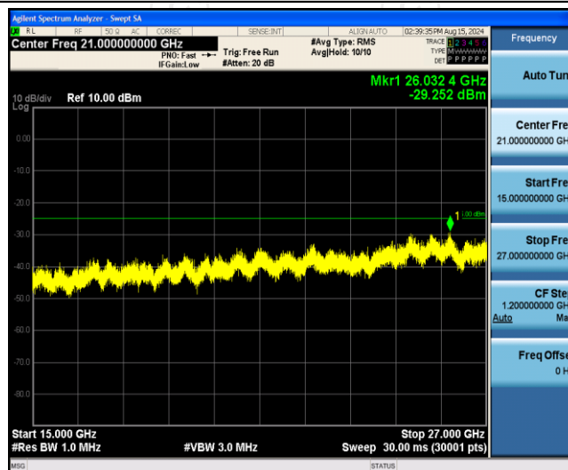
Band7-5MHz-QPSK-21425-1RB#0-Range3:15000~27000MHz
