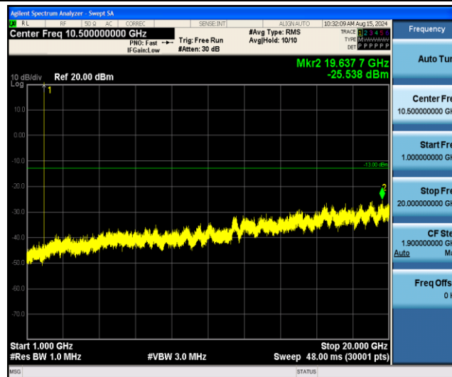
Band2-3MHz-16QAM-19185-1RB#0-Range2:1000~20000MHz
