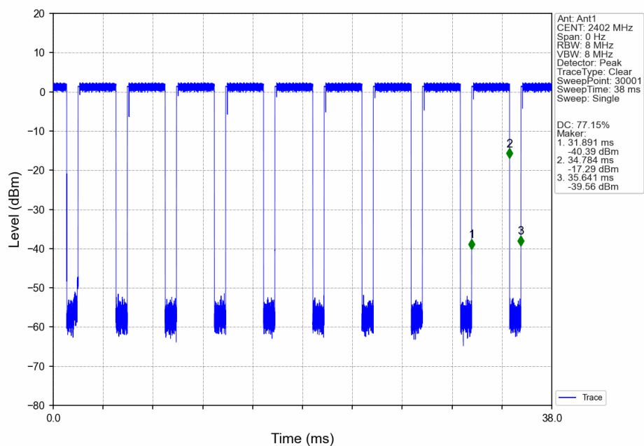
\pi/4 QPSK 2DH5 LCH 2402MHz Ant1 NTN
