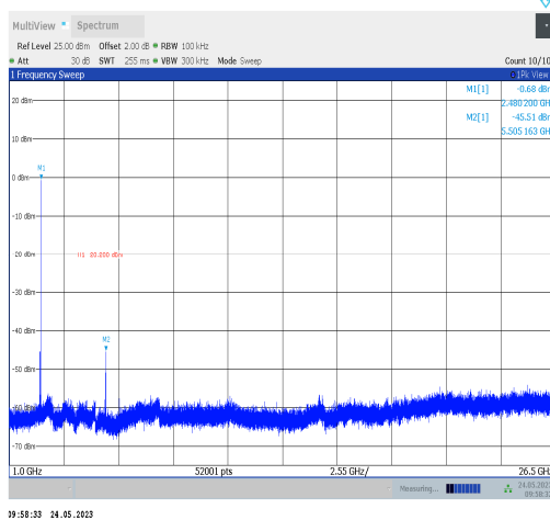
BLE_1M-Ant0-2480-1000~26500
