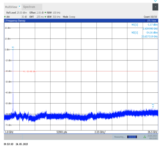
BLE_1M-Ant0-2440-1000~26500
