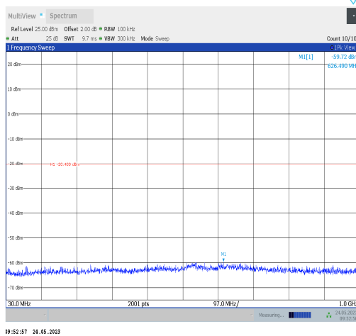
BLE_1M-Ant0-2440-30~1000
