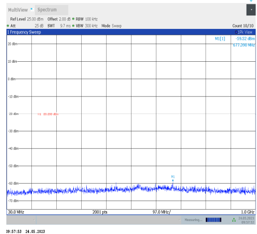
BLE_1M-Ant0-2480-30~1000
