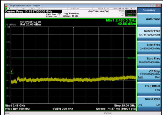
,Plot 4,2483.5MHz~25000MHz-802.11n(HT40),2452MHz,Ant0
