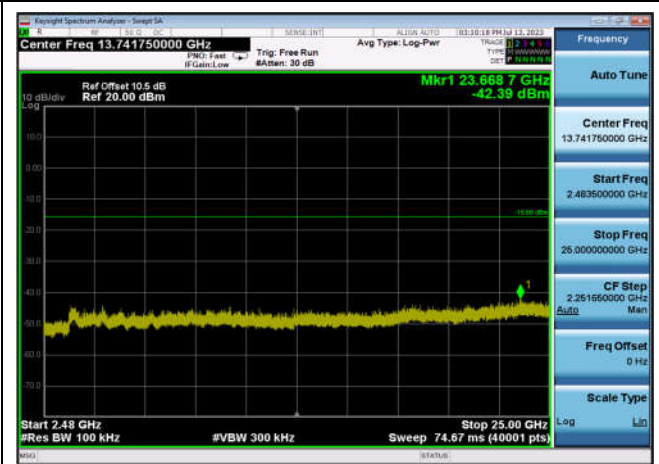
,Plot 4,2483.5MHz~25000MHz-802.11n(HT20),2462MHz,Ant0
