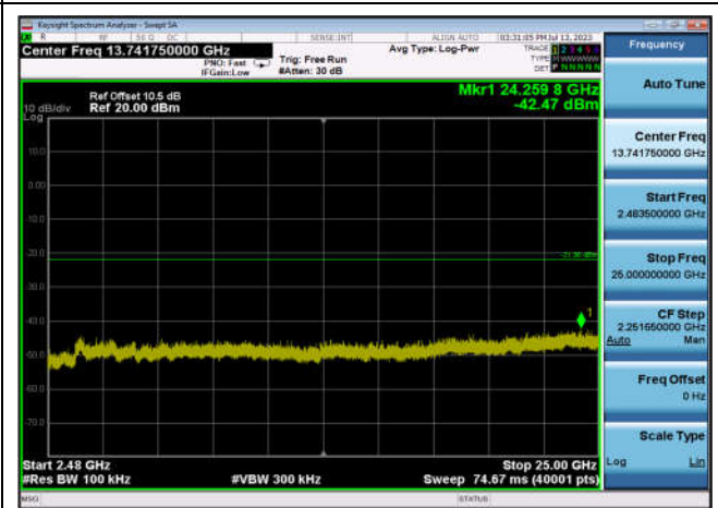
,Plot 4,2483.5MHz~25000MHz-802.11n(HT40),2452MHz,Ant0
