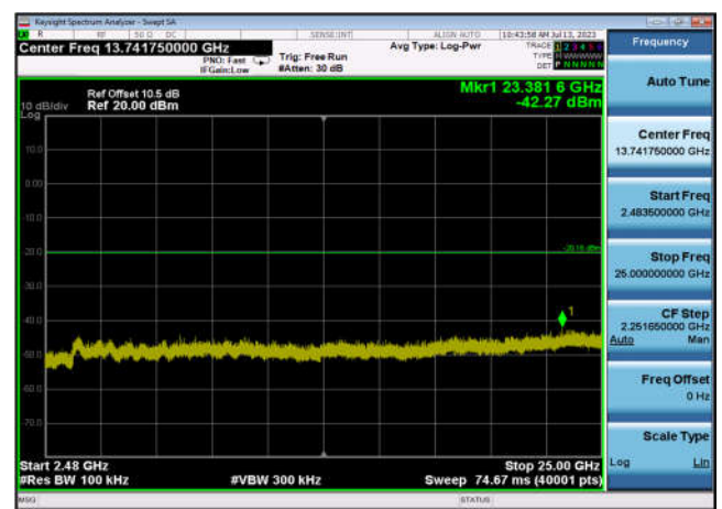
,Plot 4,2483.5MHz~25000MHz-802.11n(HT40),2452MHz,Ant0
