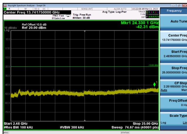
,Plot 4,2483.5MHz~25000MHz-802.11n(HT40),2452MHz,Ant0
