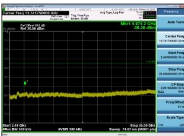
,Plot 4,2483.5MHz~25000MHz-802.11b ,2437MHz,Ant0
