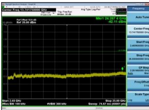
,Plot 4,2483.5MHz~25000MHz-802.11g ,2437MHz,Ant0
