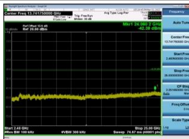
,Plot 4,2483.5MHz~25000MHz-802.11n(HT40),2452MHz,Ant0
