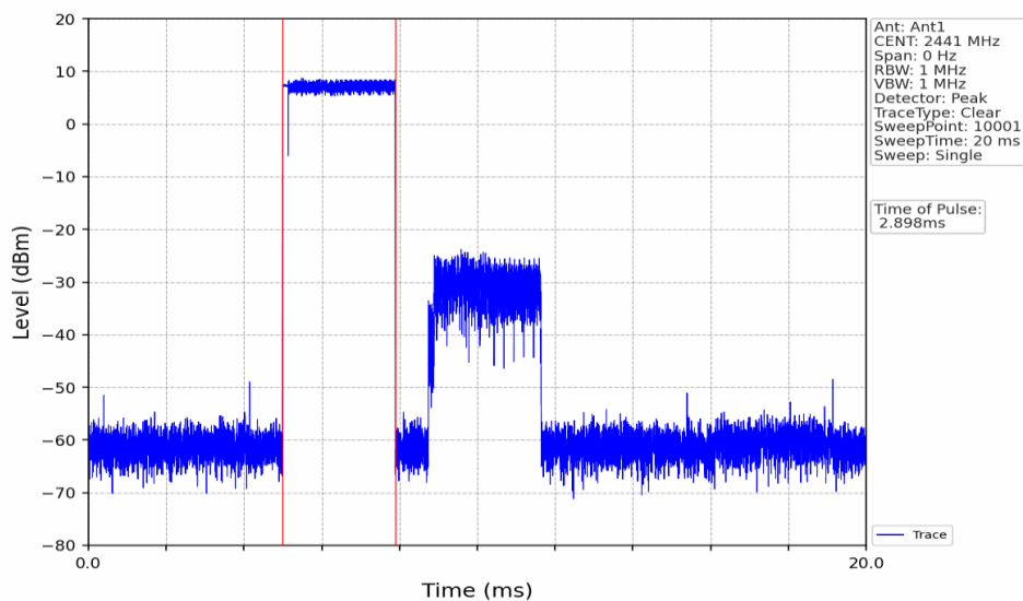
8DPSK_3DH5_HOPP_Ant1_NTNV
