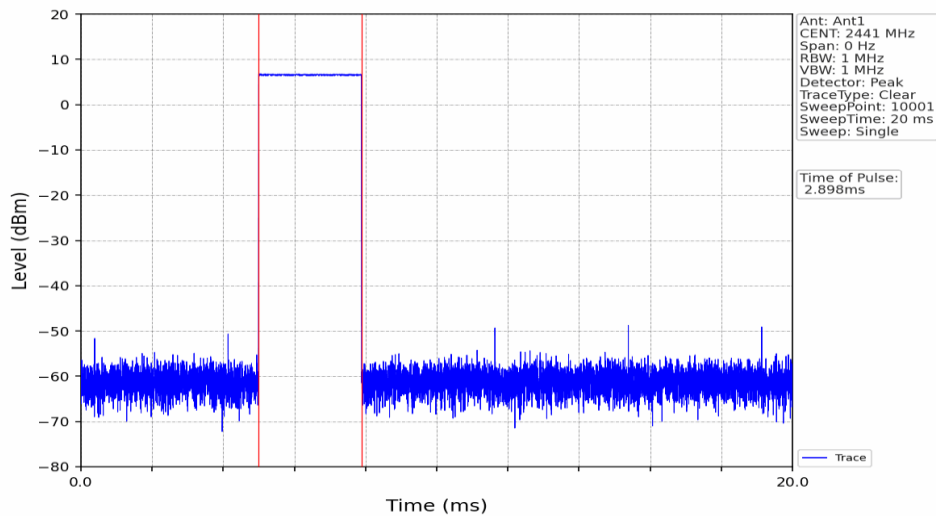
GFSK_DH5_HOPP_Ant1_NTNV
