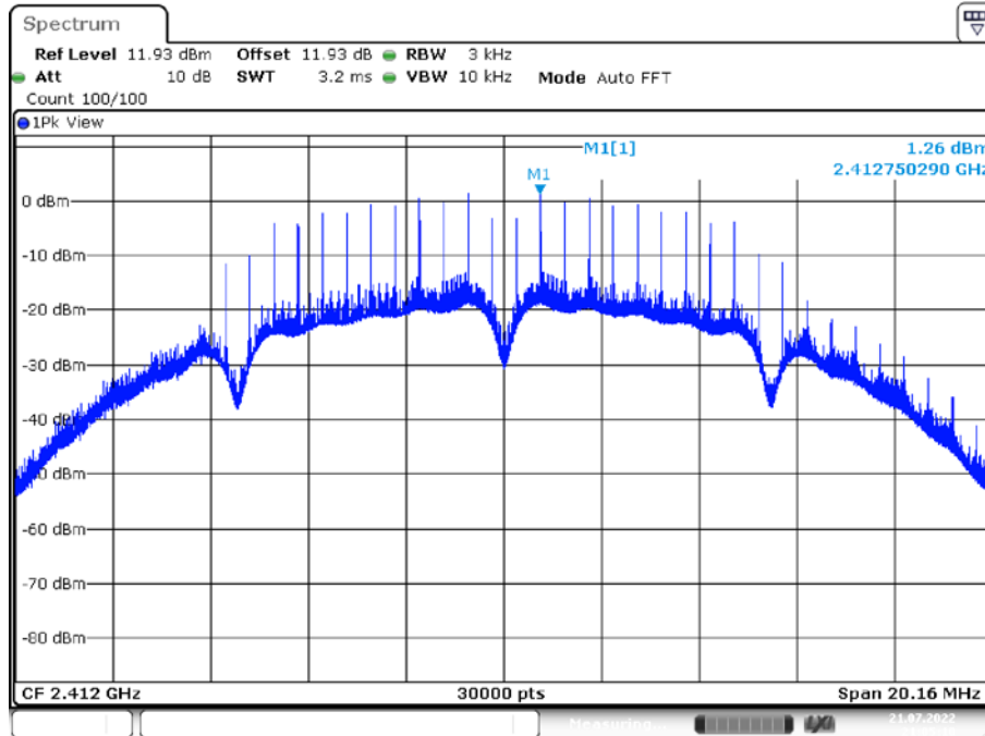
11B MIMO_Ant2_2412
