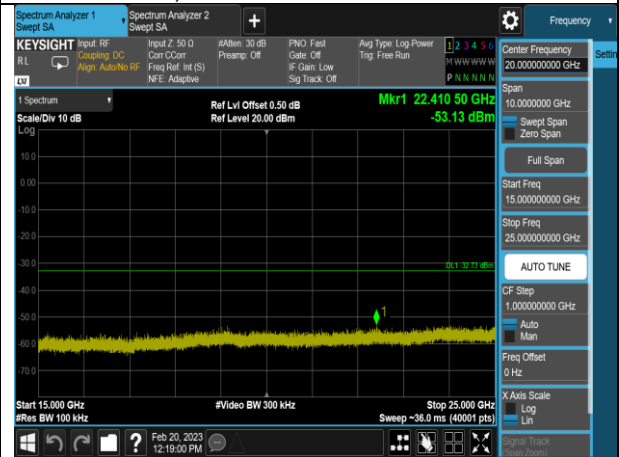
802.11n(HT40),2452MHz,Ant0,Plot 6,15000MHz~25000MHz
