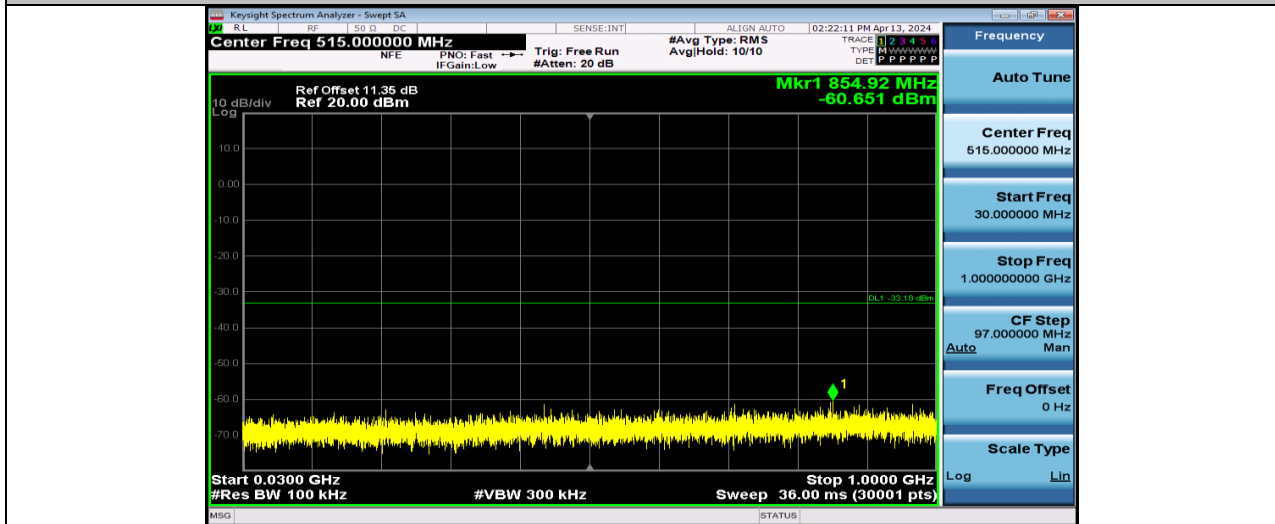
11G-Ant1-2412-30~1000-PASS
