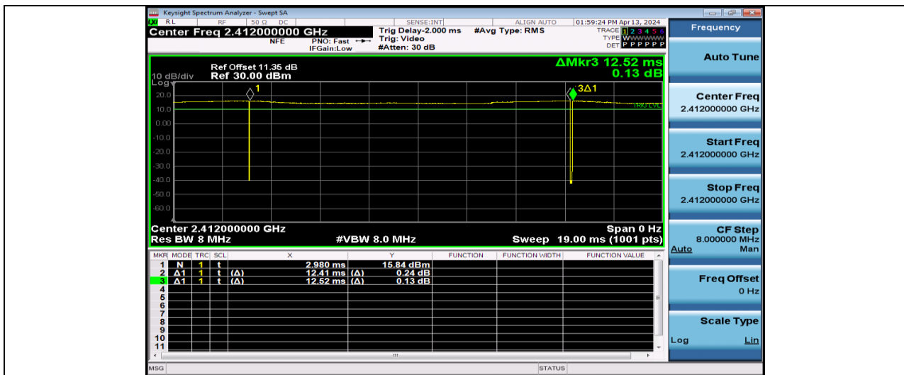
NTVN-11B-Ant1-2412
