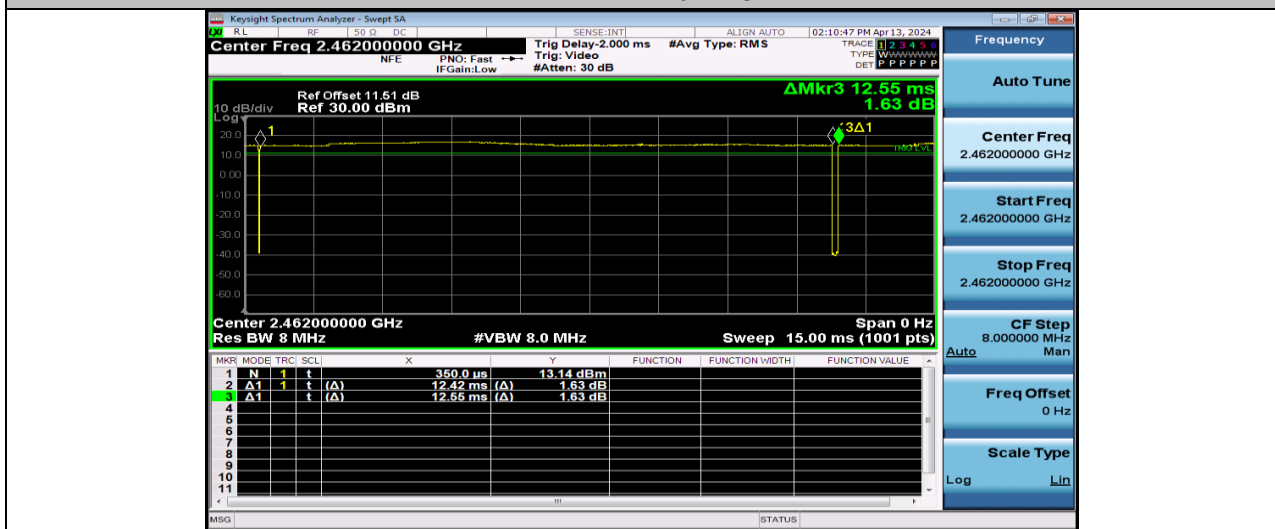
NTVN-11B-Ant1-2462
