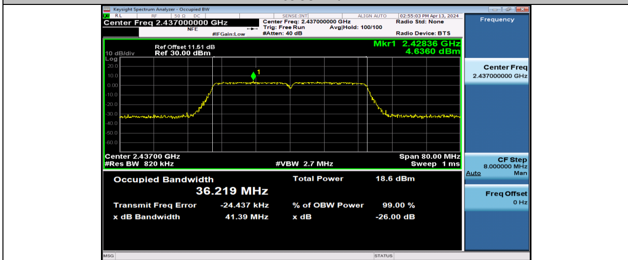
11N40ISO-Ant1-2437
