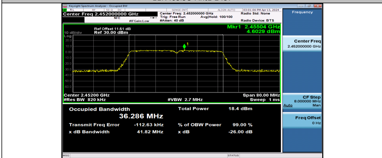
11N40ISO-Ant1-2452
