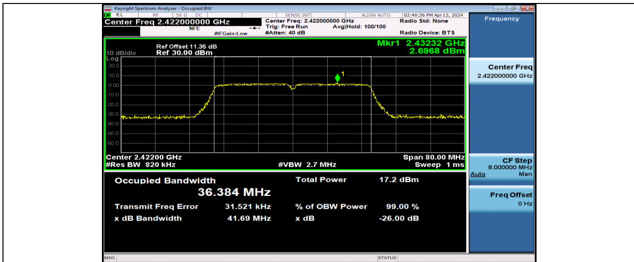
11N40ISO-Ant1-2422
