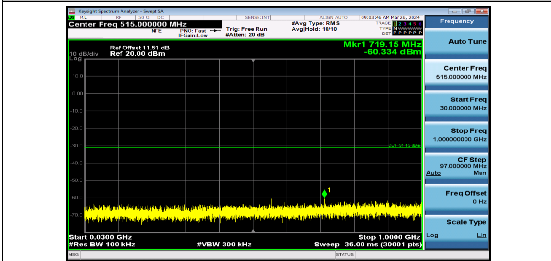
11G-Ant1-2462-30~1000-PASS
