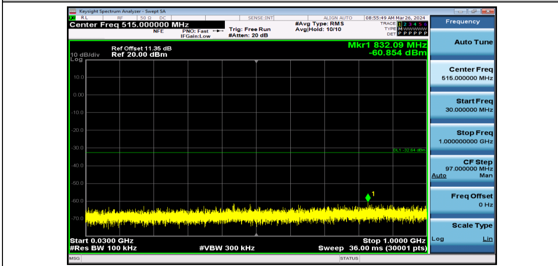
11G-Ant1-2412-30~1000-PASS
