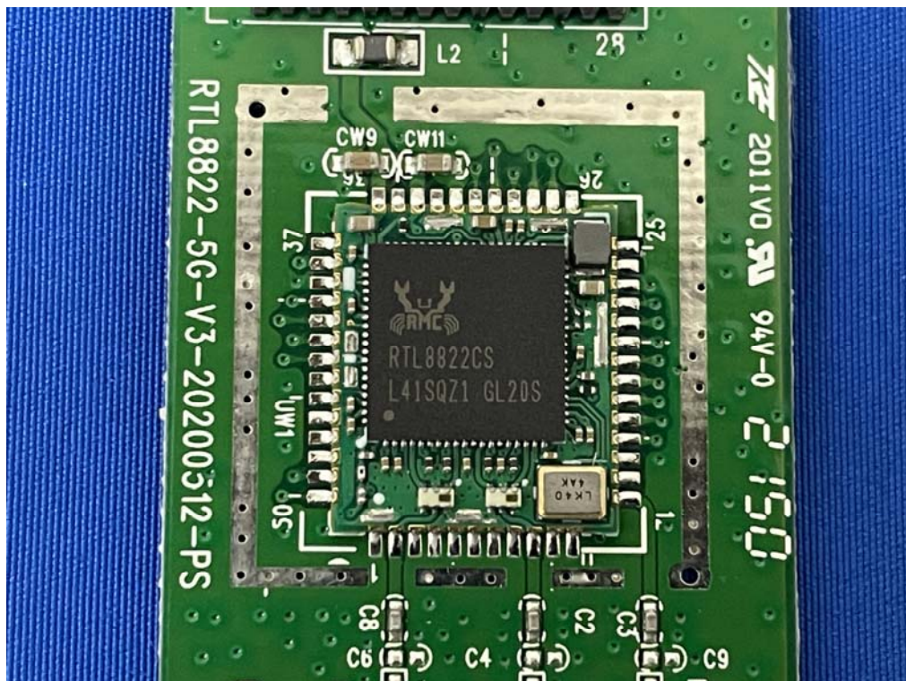
<BT/WIFI Module>
