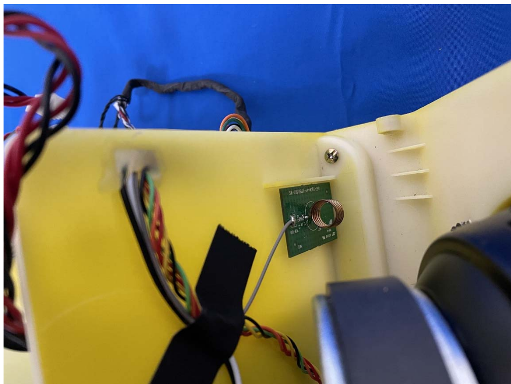
<UHF_Antenna>
