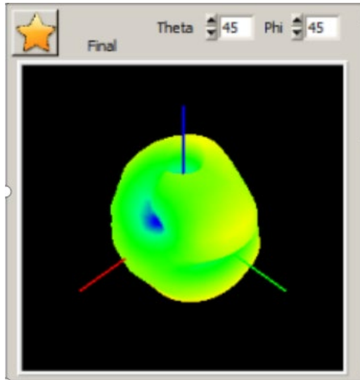
GSM900 -TRP
