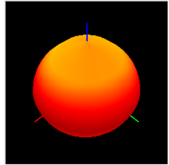
GSM850 -TIS
