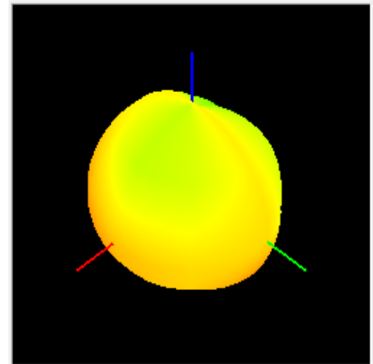
GSM900 -TIS
