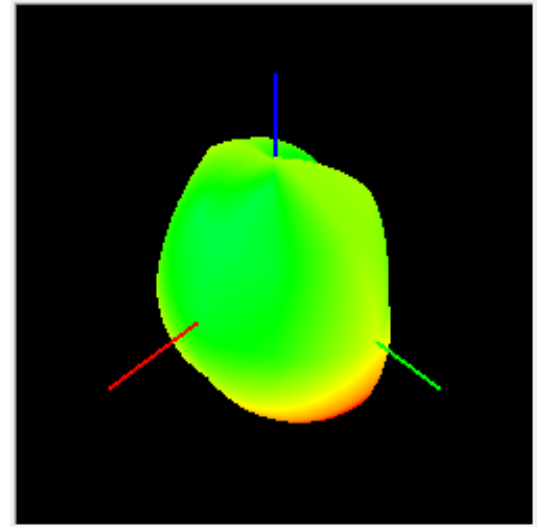
W2-TIS
