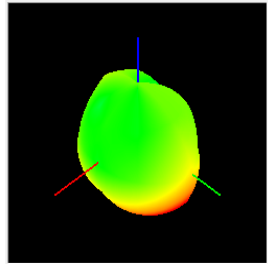
PCS1900 -TIS
