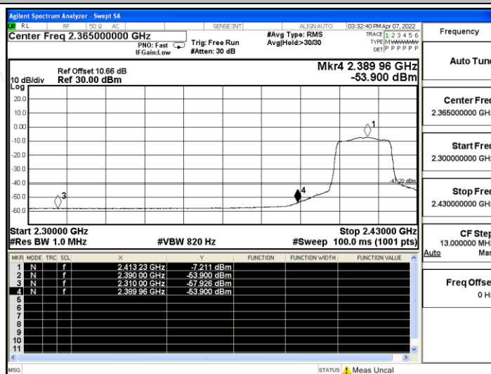
11AX20SISO_Ant B_Low_2412_AV
