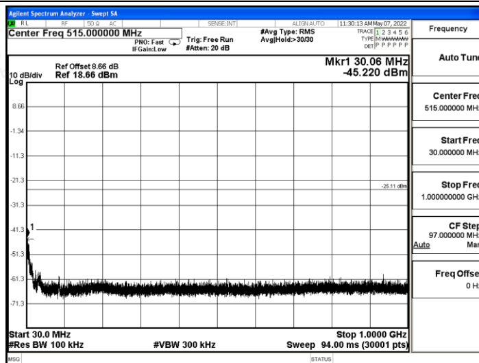
11AX20SISO_Ant B_2412_30~1000
