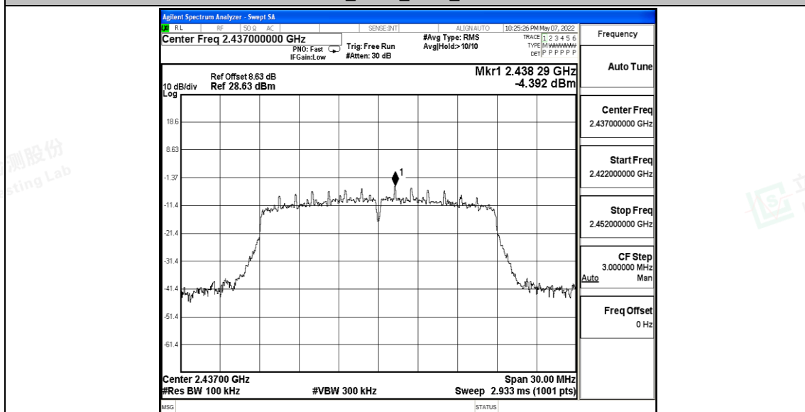
11N20SISO_Ant B_2437_30~1000
