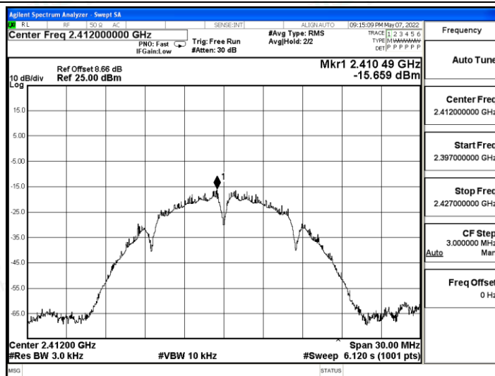
11B_Ant B_2437
