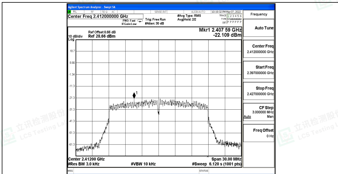
11AX20SISO_Ant B_2437
