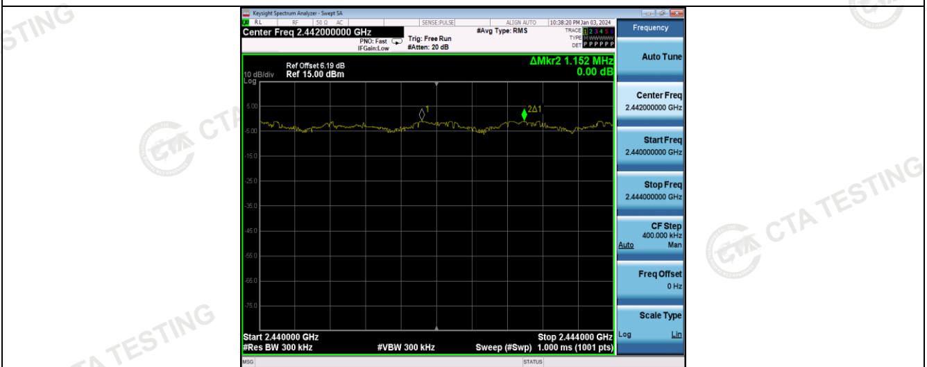
8DPSK
