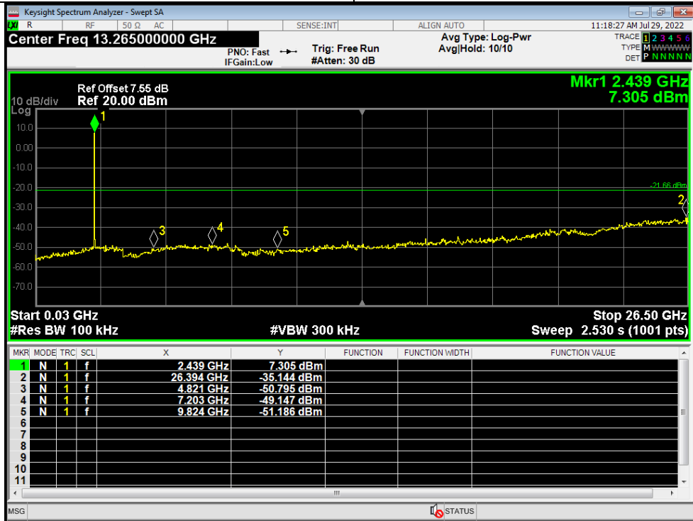
0.03GHz~26.5GHz
