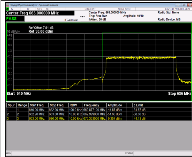
Band71-20MHz-16QAM-133372-1RB#99
