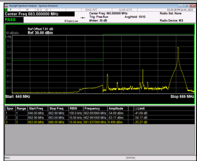
Band71-20MHz-16QAM-133372-1RB#0
