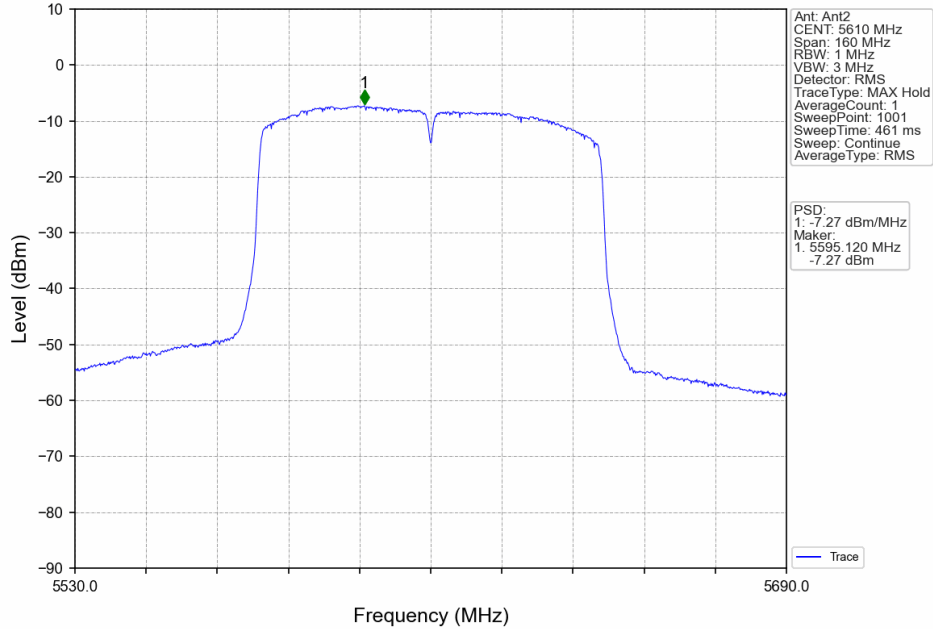
802.11ac(VHT80)_HCH_5610MHz_MIMO_NTNV
