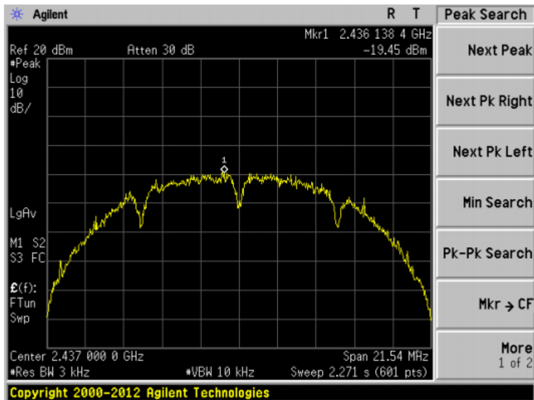
802.11b-2437MHz
