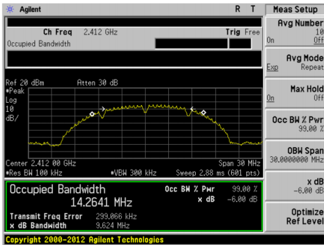
802.11b-CH2412MHZ
