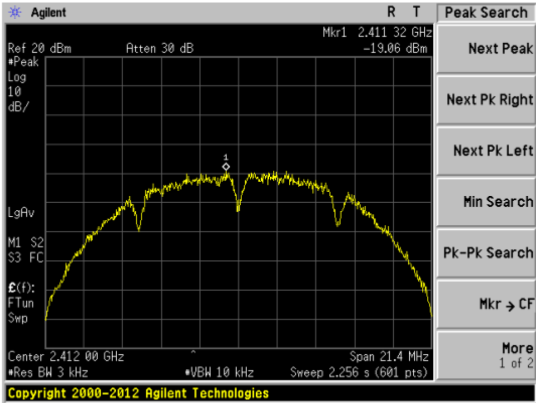
802.11b-2412MHz
