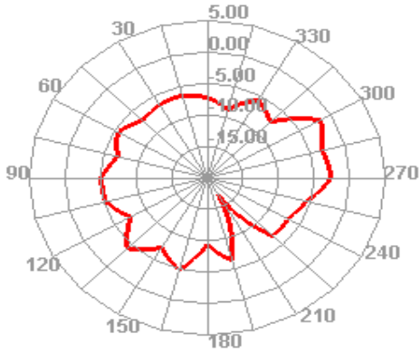
2450.000MHz E1
