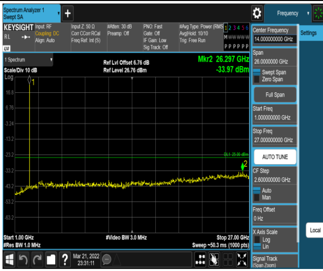
Band38-20MHz-QPSK-37850-1RB#0-Range2:1000~27000MHz
