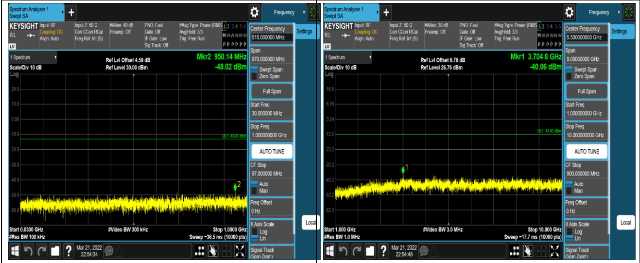
Band13-5MHz-QPSK-23255-1RB#0-Range1:30~1000MHz
