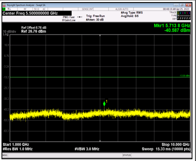
Band12-1.4MHz-QPSK-23017-1RB#0-Range2:1000~10000MHz
