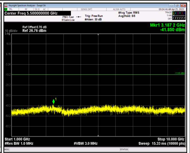
Band13-5MHz-QPSK-23255-1RB#0-Range2:1000~10000MHz
