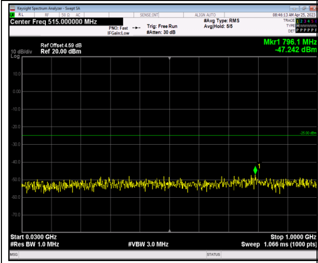
Band12-1.4MHz-QPSK-23017-1RB#0-Range1:30~1000MHz
