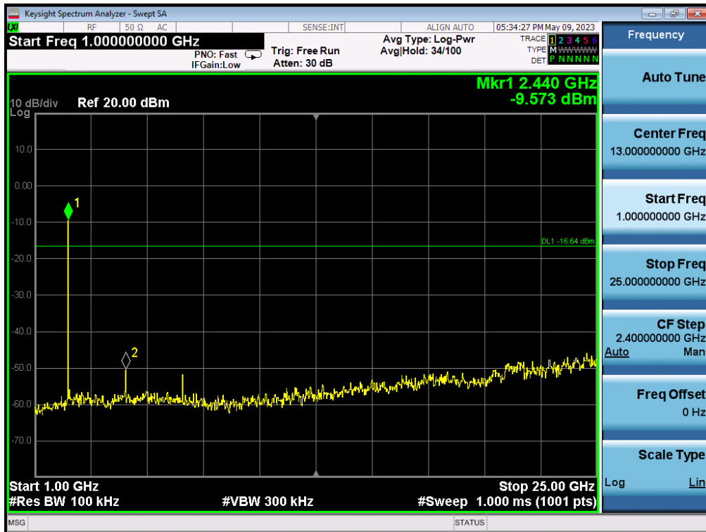
1GHz-25GHz
