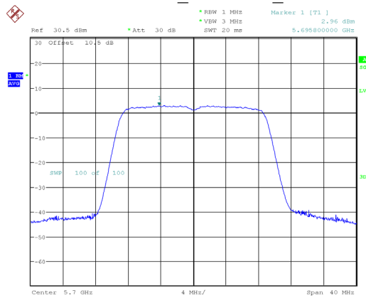
802.11ac20_5700MHz_Chain 1
