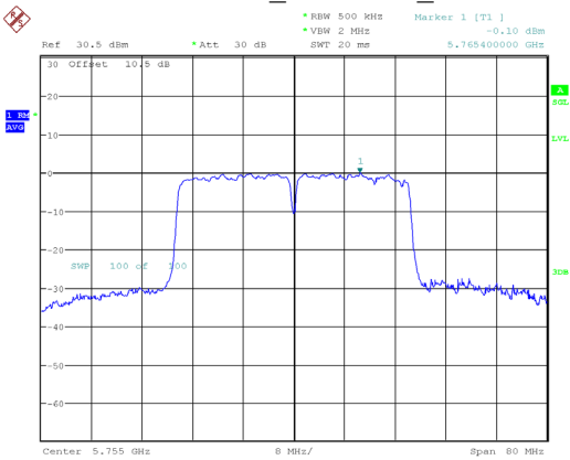
802.11ac40_5755MHz_Chain 0
