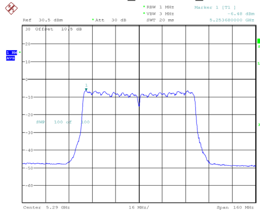
802.11ac80_5290MHz_Chain 1
