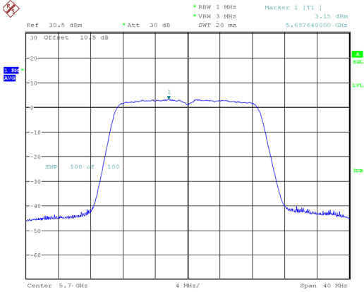
802.11ac20_5700MHz_Chain 0
