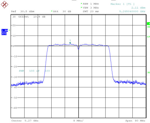
802.11ac40_5270MHz_Chain 1
