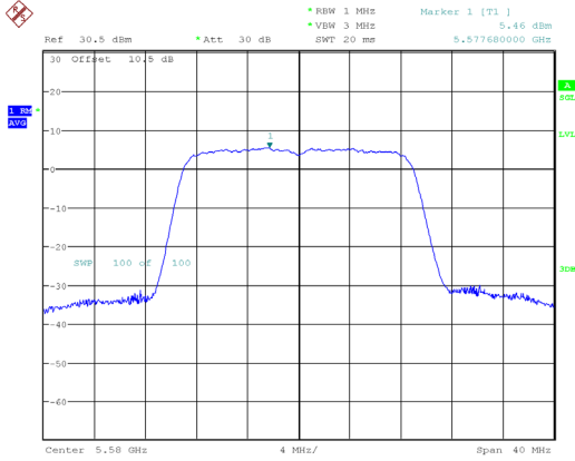
802.11ac20_5580MHz_Chain 0
