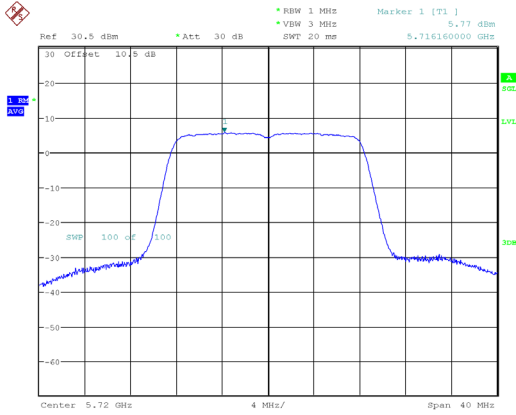
802.11a_5720MHz_Chain 1
