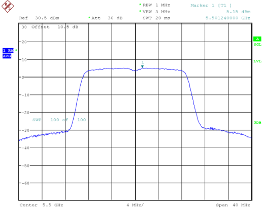
802.11ac20_5500MHz_Chain 0
