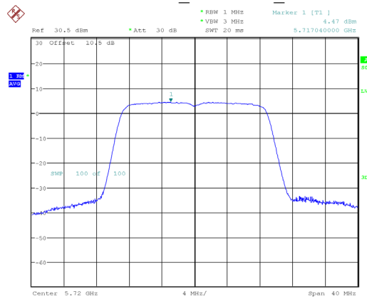
802.11ac20_5720MHz_Chain 1
