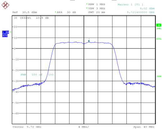
802.11a_5720MHz_Chain 0
