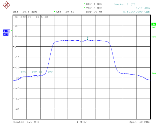
802.11a_5500MHz_Chain 1
