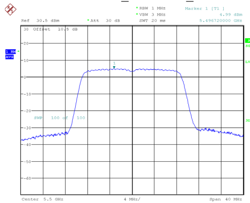
802.11ac20_5500MHz_Chain 1
