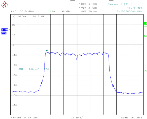
802.11ac80_5290MHz_Chain 0
