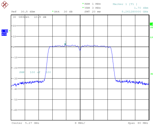
802.11ac40_5270MHz_Chain 0
