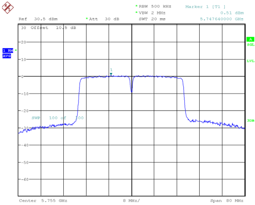
802.11ac40_5755MHz_Chain 1
