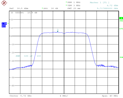
802.11ac20_5720MHz_Chain 0
