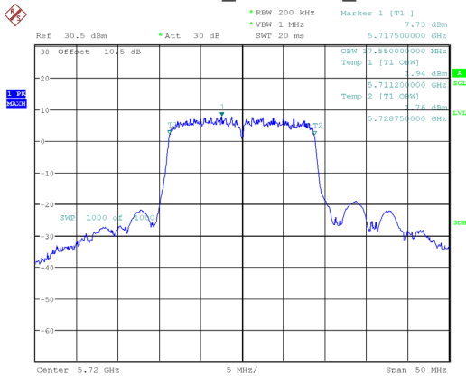
802.11ac20_5720MHz_Chain 0
