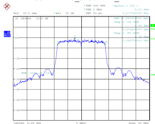
802.11ac20_5280MHz_Chain 1
