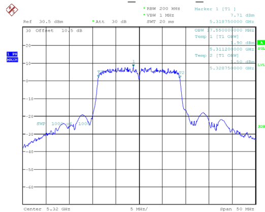
802.11ac20_5320MHz_Chain 0
