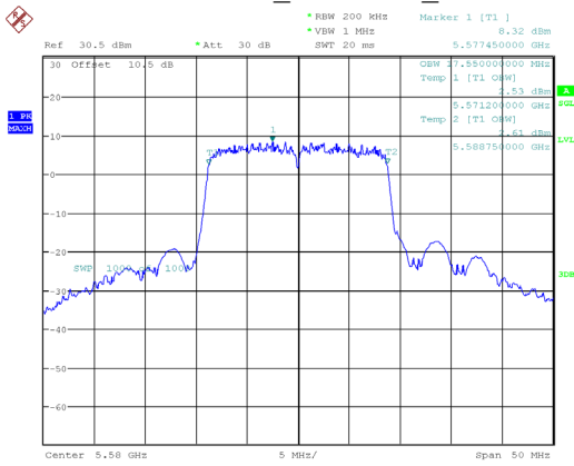
802.11ac20_5580MHz_Chain 0
