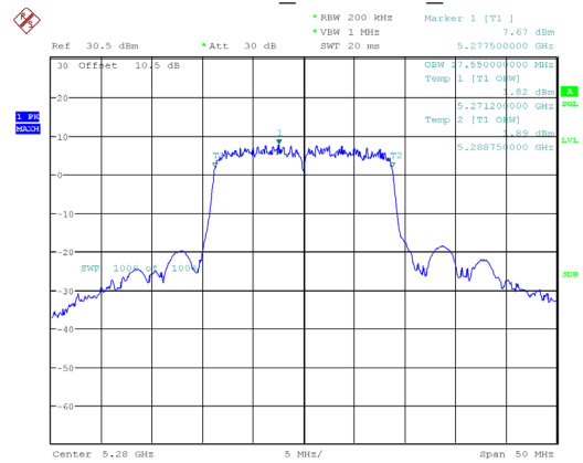
802.11ac20_5280MHz_Chain 0
