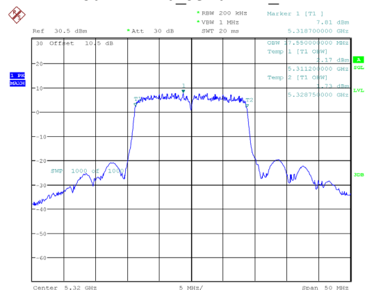
802.11ac20_5320MHz_Chain 1
