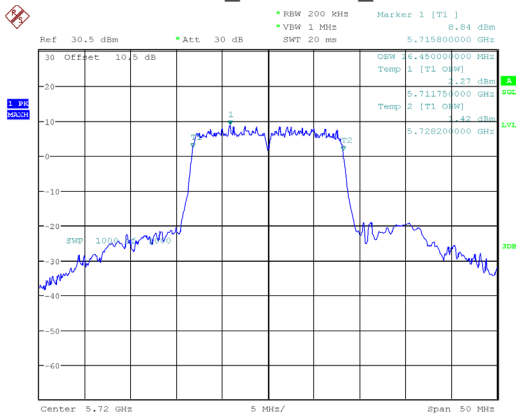
802.11a_5720MHz_Chain 1
