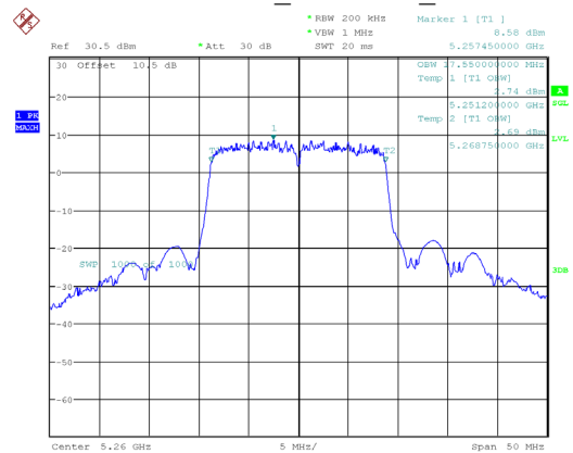
802.11ac20_5260MHz_Chain 1
