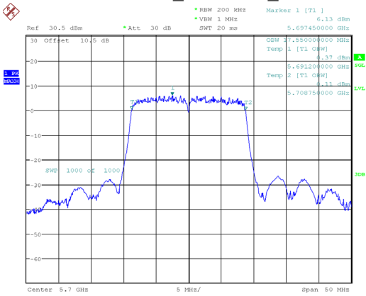
802.11ac20_5700MHz_Chain 0
