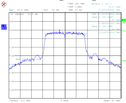
802.11ac20_5500MHz_Chain 0
