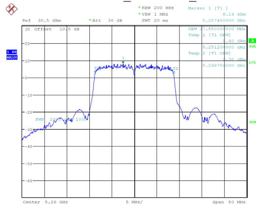
802.11ac20_5260MHz_Chain 0
