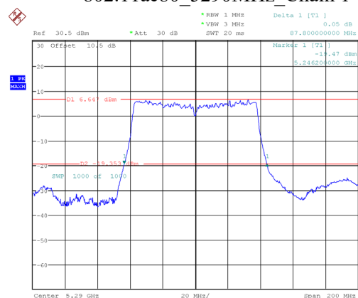
802.11ac80 5290MHz Chain 1
