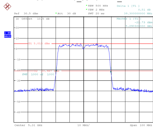
802.11ac40 5310MHz Chain 1
