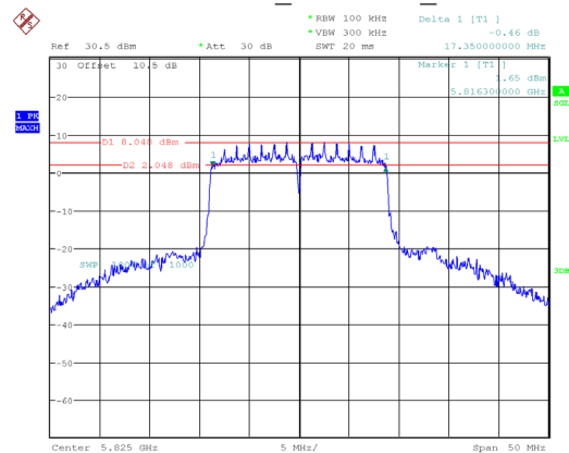
802.11ac20 5825MHz Chain 1
