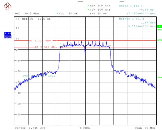
802.11ac20 5745MHz Chain 1
