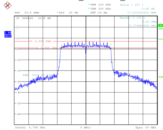
802.11ac20_5785MHz_Chain 0
