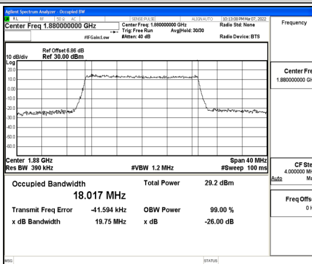
Band2-20MHz-QPSK-19100-100RB#0
