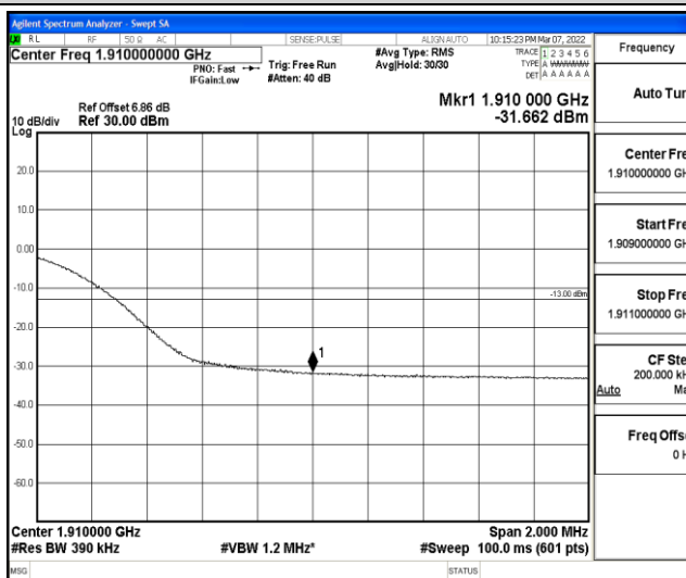
Band2-20MHz-16QAM-19100-100RB#0
