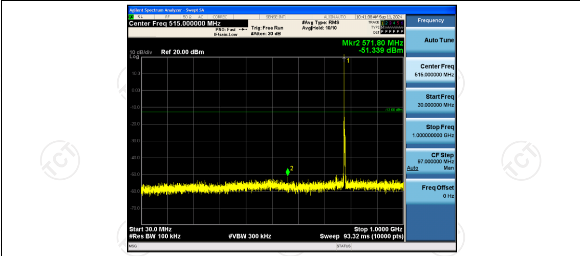
Band13-5MHz-QPSK-23230-1RB#0-Range1:30~1000MHz
