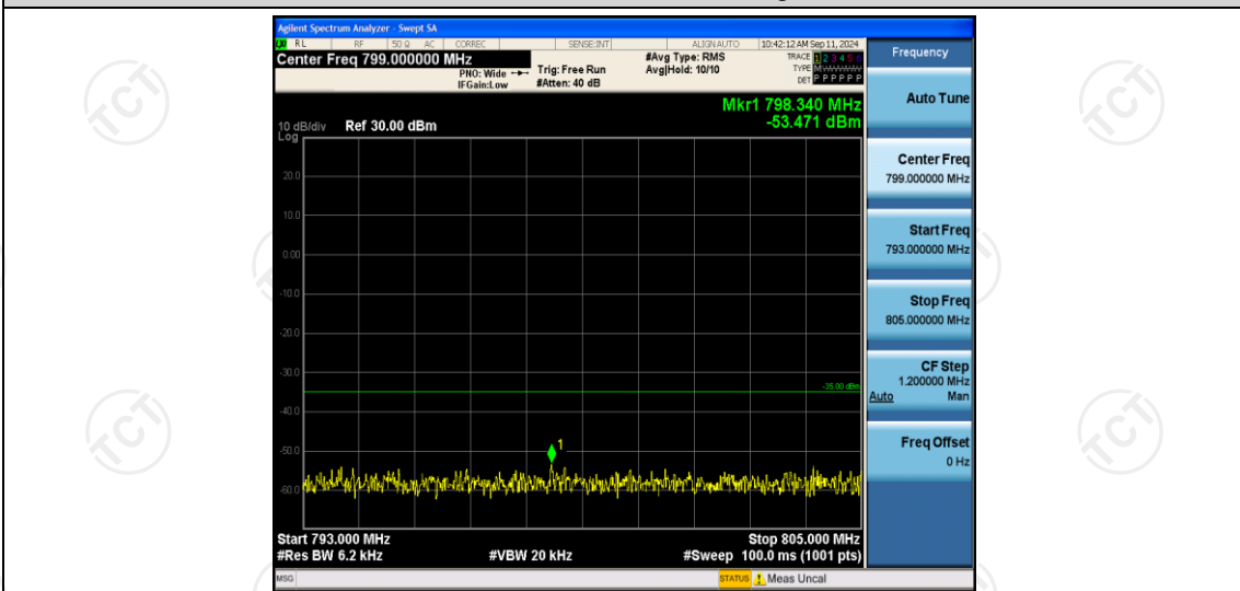
Band13-5MHz-QPSK-23230-1RB#0-Range4:793~805MHz
