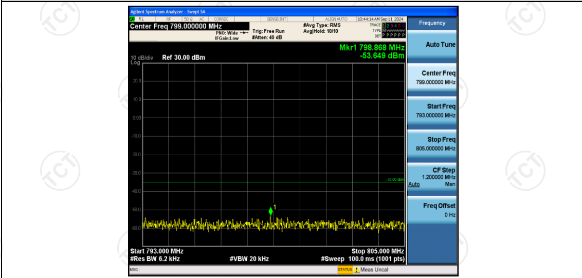
Band13-5MHz-QPSK-23255-1RB#0-Range4:793~805MHz
