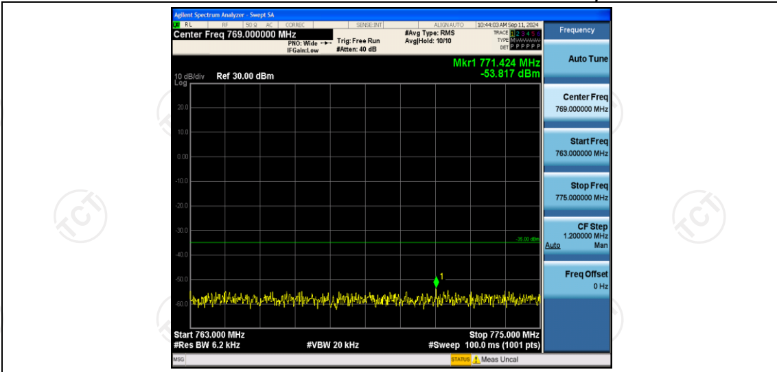
Band13-5MHz-QPSK-23255-1RB#0-Range3:763~775MHz
