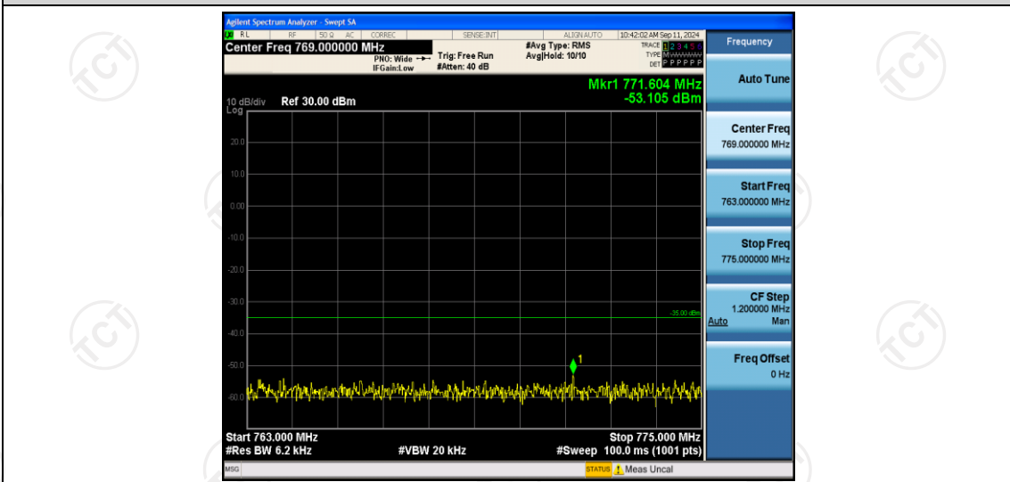
Band13-5MHz-QPSK-23230-1RB#0-Range3:763~775MHz
