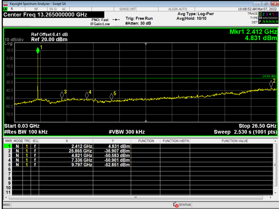
0.03GHz~26.5GHz
