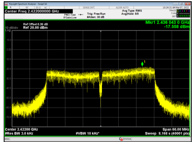
2422MHz
