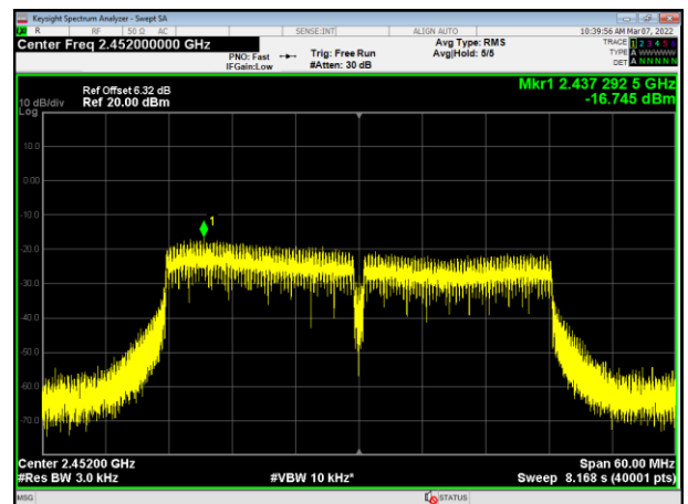
2452MHz
