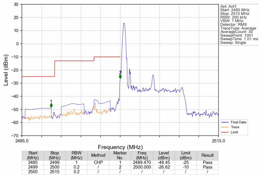
Band7_10MHz_QPSK_LCH_2505MHz_RB_1_0_NTNV
