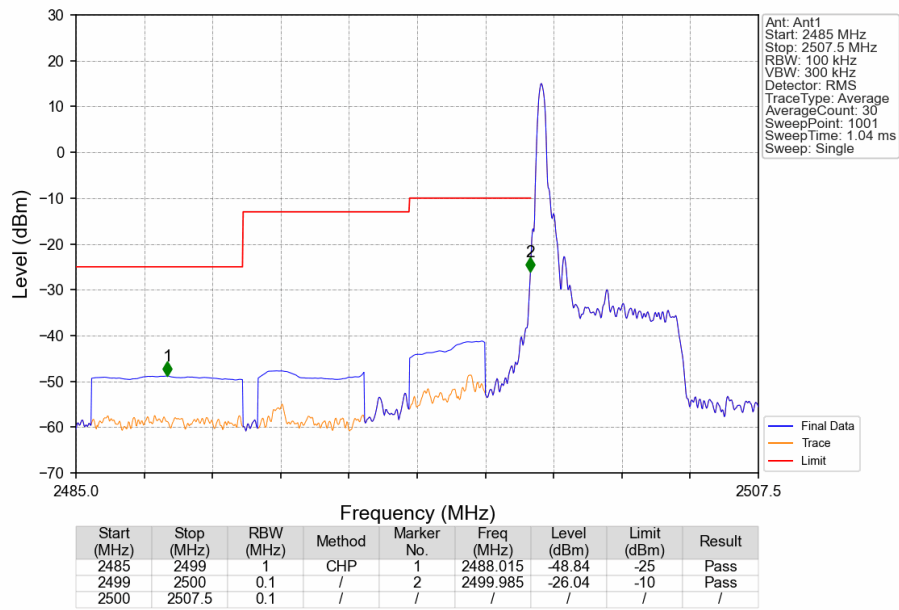
Band7_5MHz_QPSK_LCH_2502.5MHz_RB_1_0_NTNV
