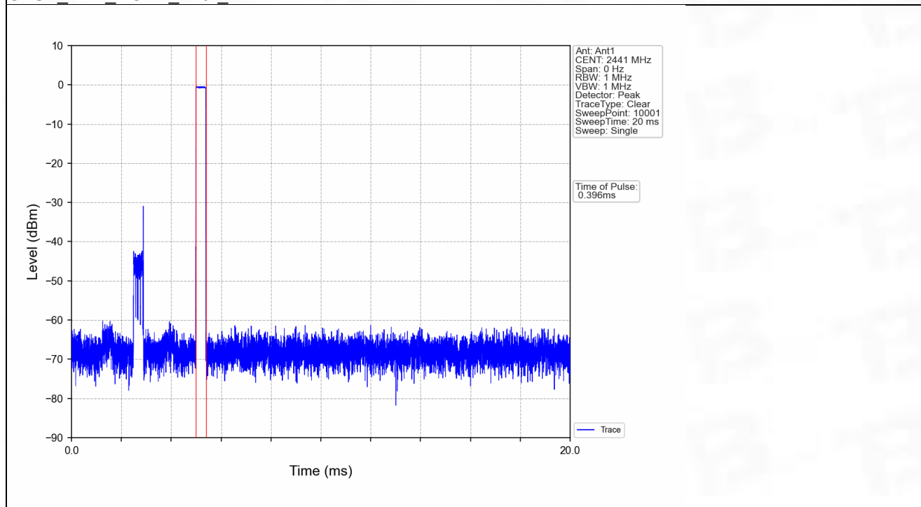
GFSK_DH1_HOPP_Ant1_NTNV
