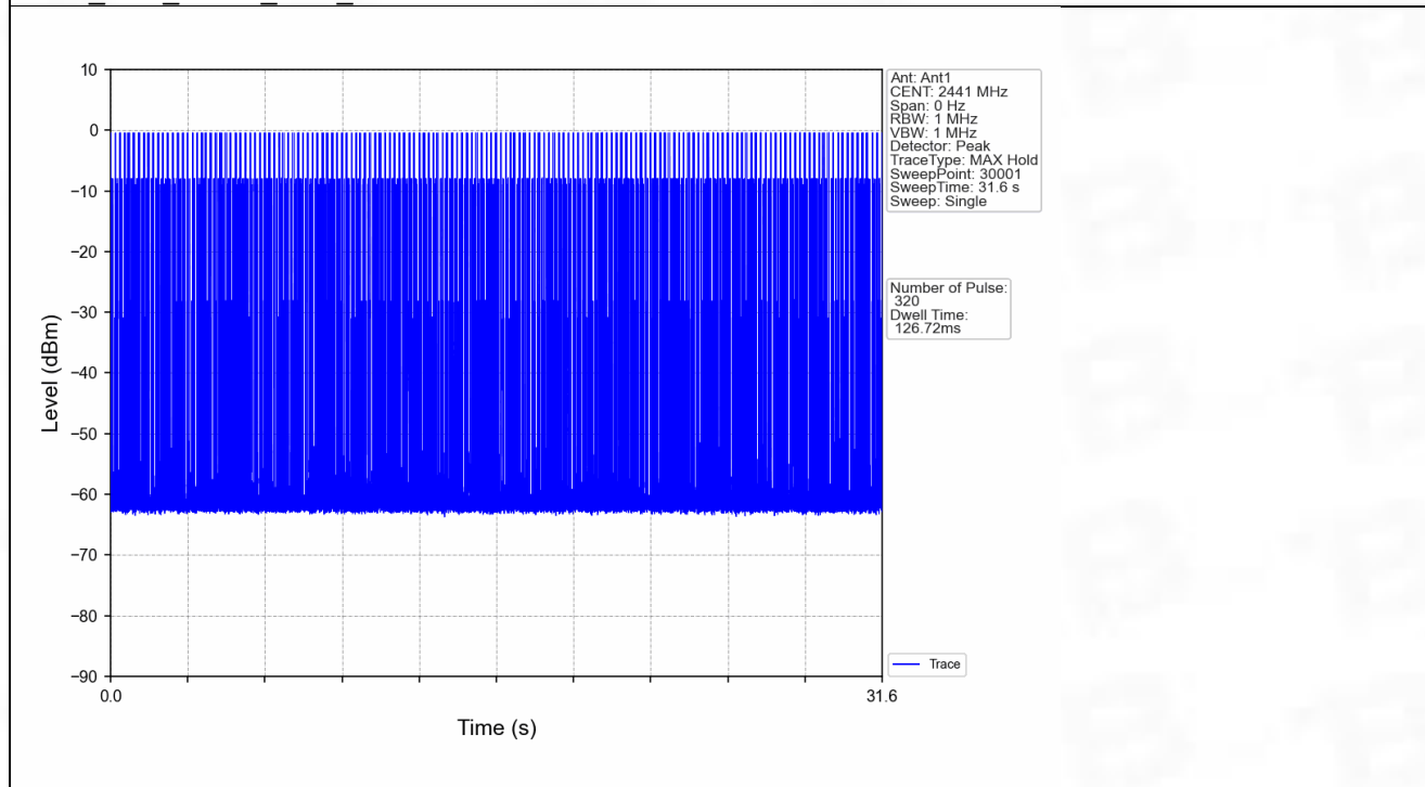
GFSK_DH1_HOPP_Ant1_NTNV
