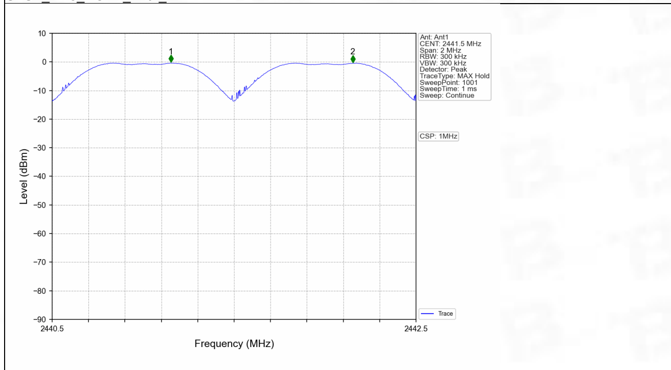
Pi/4DQPSK_2DH5_HOPP_Ant1_NTNV
