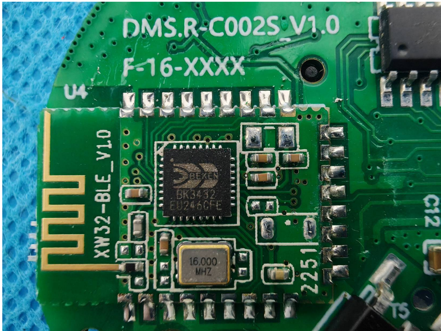
RF Module
