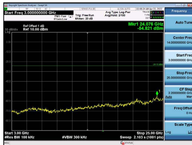
3GHz -25GHz
