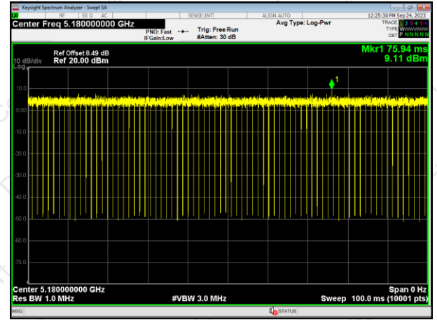
802.11n HT20
