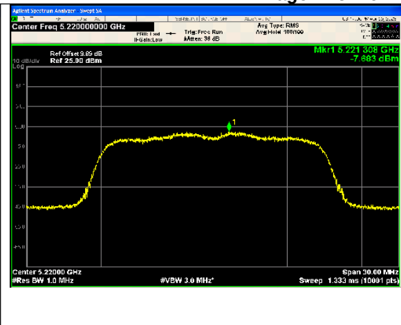
IEEE 802.11n_Channel 44_20MHz_Antenna 0
