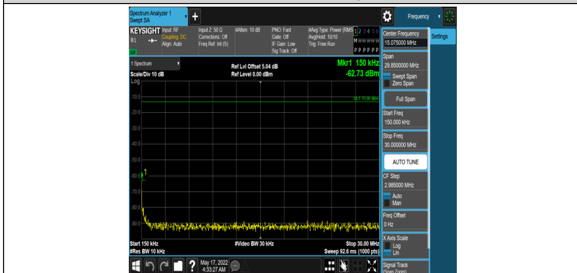
Band12-5MHz-QPSK-23095-1RB#0-Range2:0.15~30MHz
