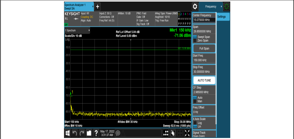
Band7-20MHz-QPSK-21100-1RB#0-Range2:0.15~30MHz
