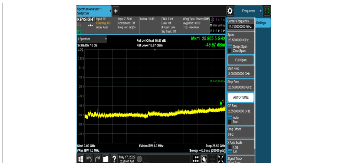
Band7-5MHz-QPSK-21425-1RB#0-Range5:3000~26500MHz
