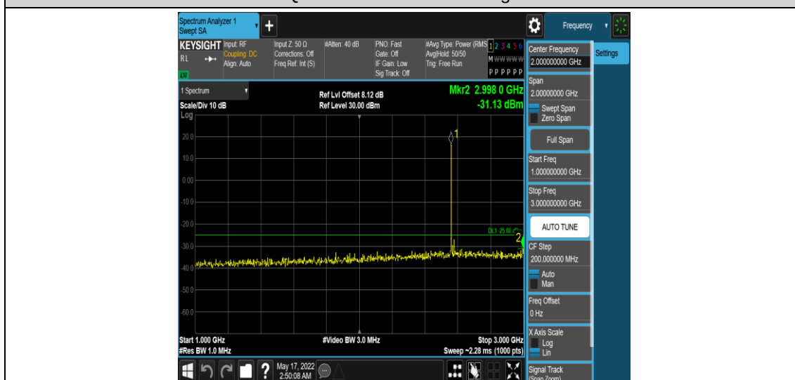
Band7-10MHz-QPSK-21400-1RB#0-Range4:1000~3000MHz
