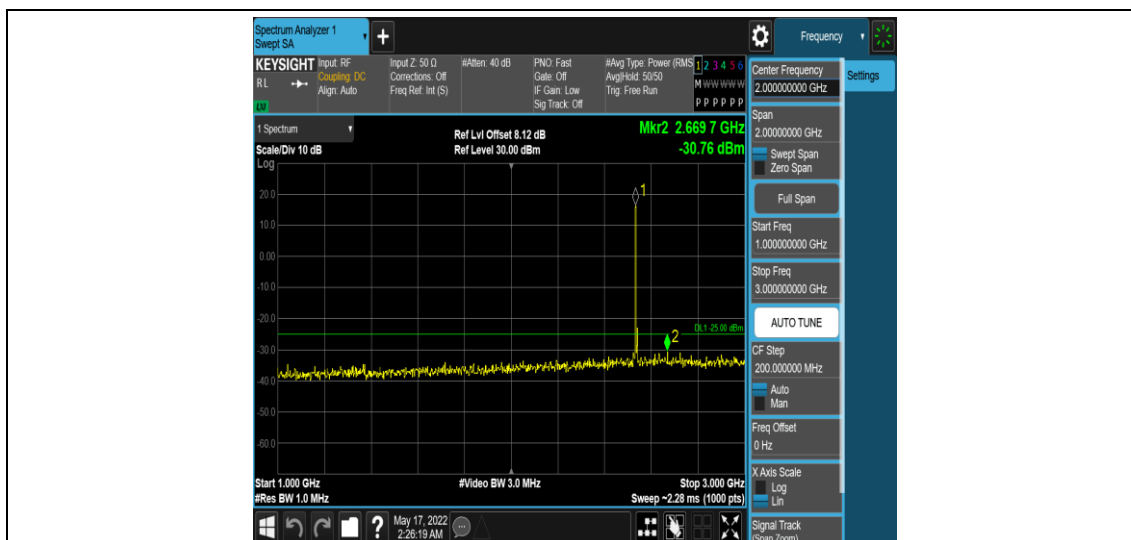
Band7-5MHz-QPSK-21100-1RB#0-Range4:1000~3000MHz
