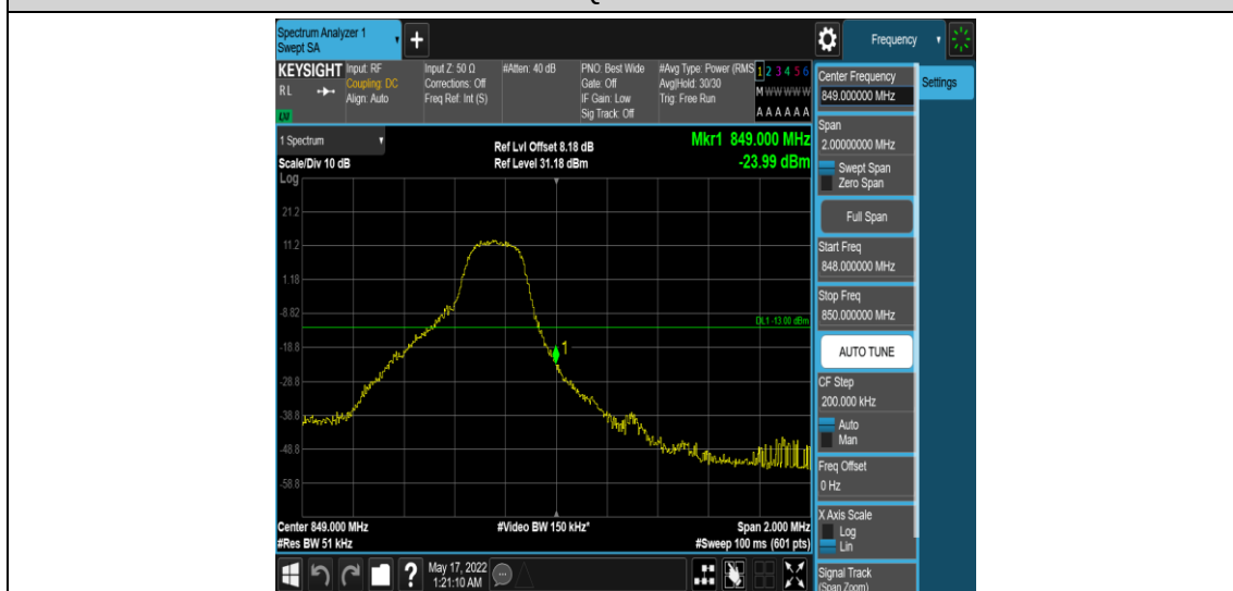
Band5-3MHz-QPSK-20635-1RB#14
