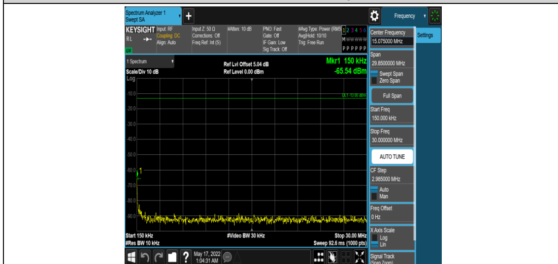
Band5-1.4MHz-QPSK-20525-1RB#0-Range2:0.15~30MHz
