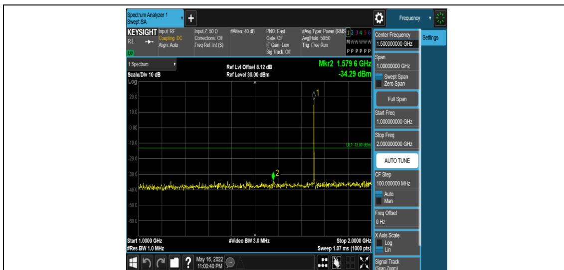
Band4-1.4MHz-QPSK-20393-1RB#0-Range4:1000~2000MHz
