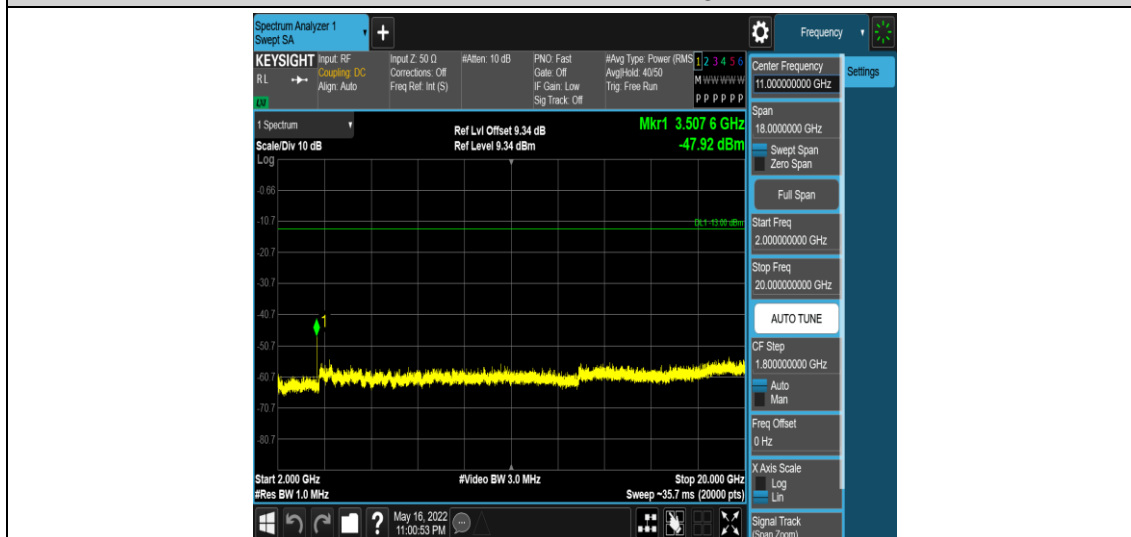
Band4-1.4MHz-QPSK-20393-1RB#0-Range5:2000~20000MHz
