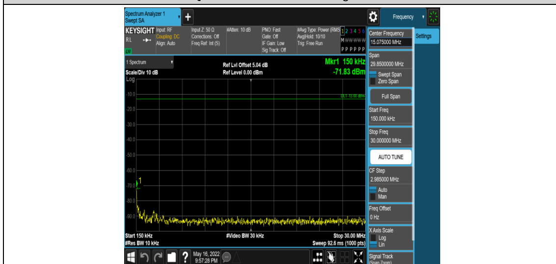
Band2-10MHz-QPSK-19150-1RB#0-Range2:0.15~30MHz
