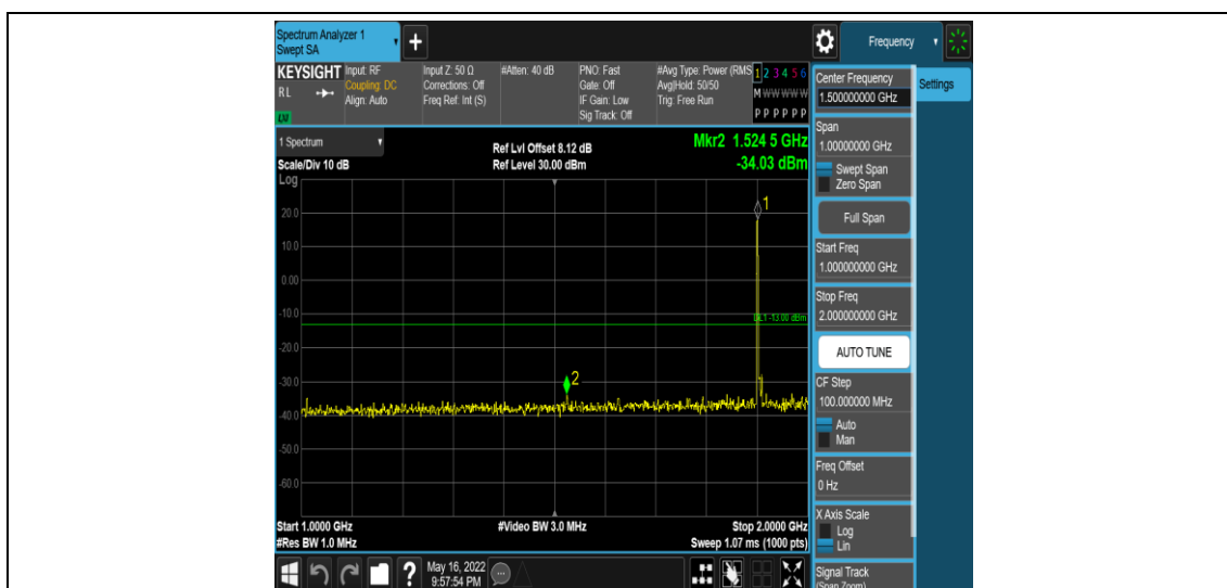
Band2-10MHz-QPSK-19150-1RB#0-Range4:1000~2000MHz
