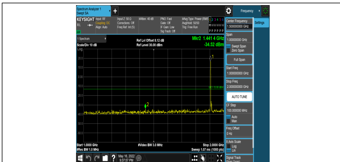
Band2-5MHz-16QAM-19175-1RB#0-Range4:1000~2000MHz
