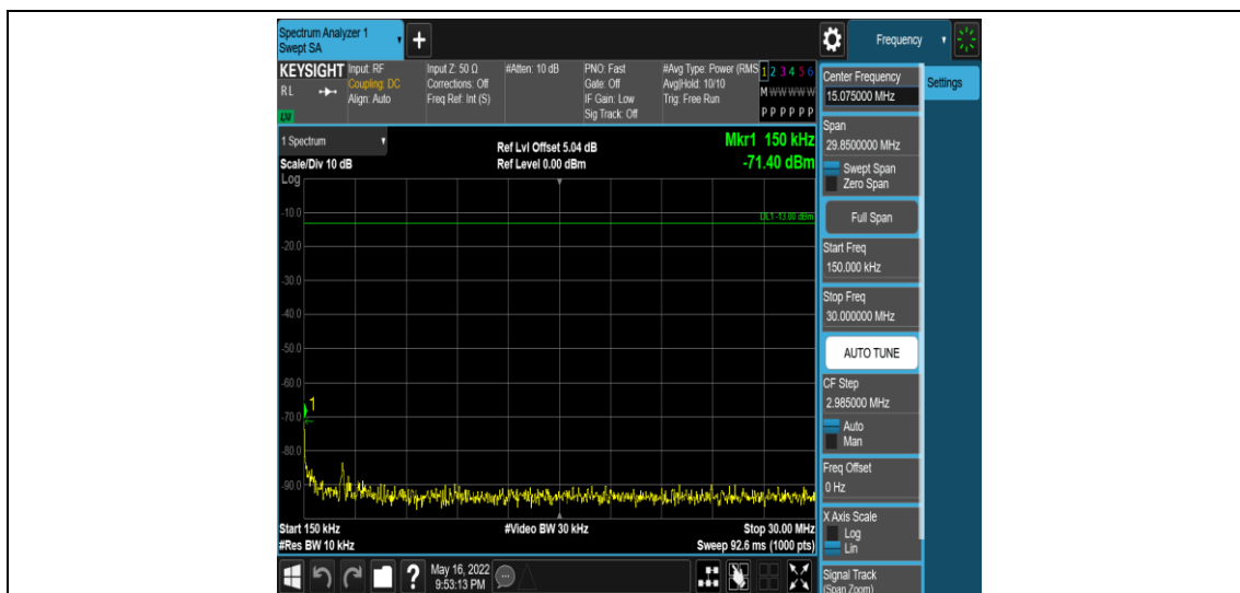
Band2-10MHz-QPSK-18650-1RB#0-Range2:0.15~30MHz
