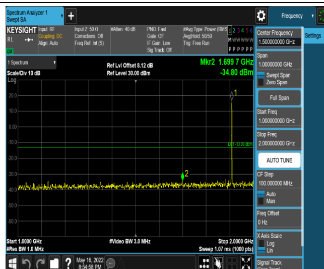
Band2-1.4MHz-QPSK-19193-1RB#0-Range4:1000~2000MHz
